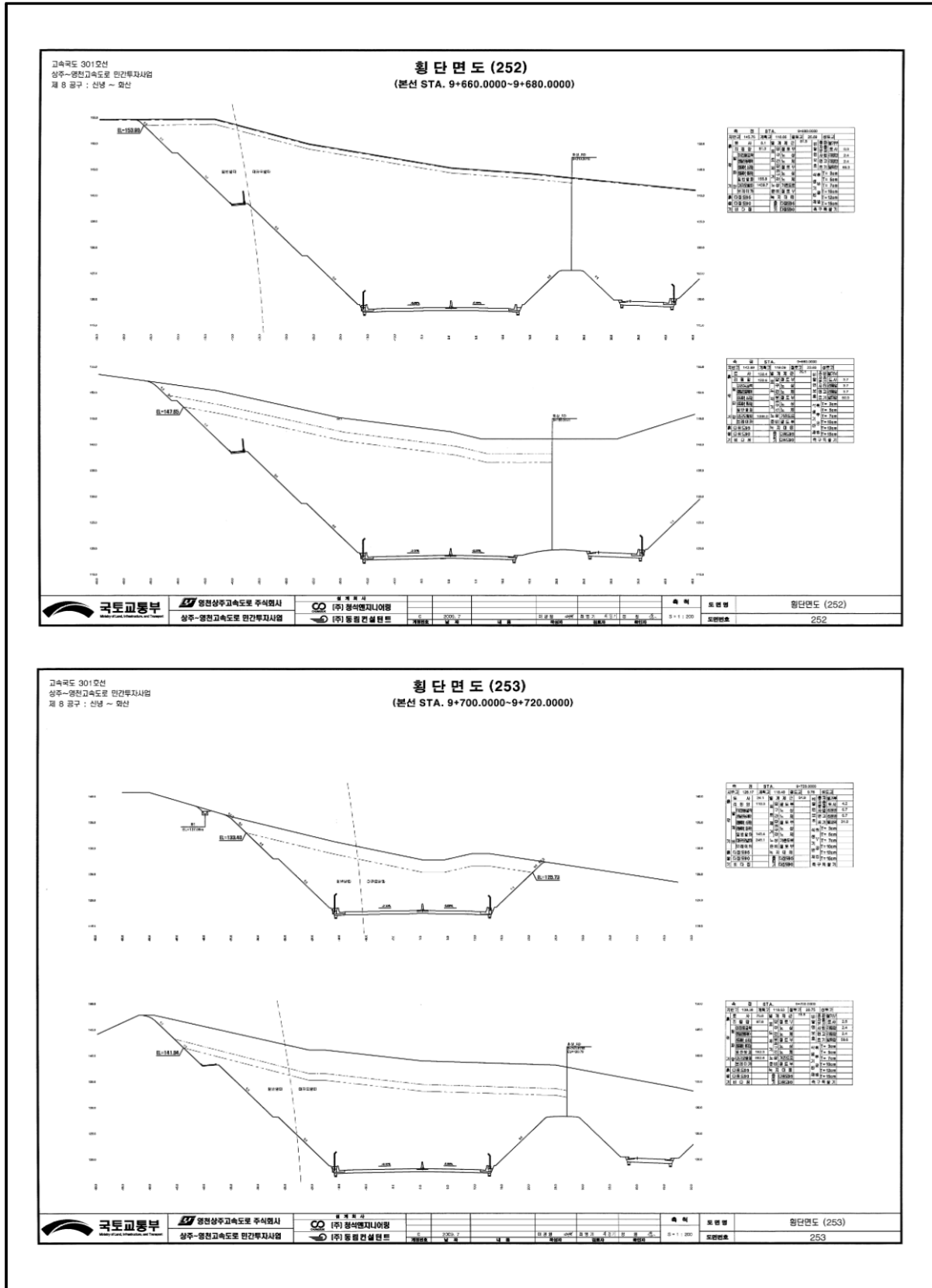
【그림 56.1.5】 표준횡단면도
